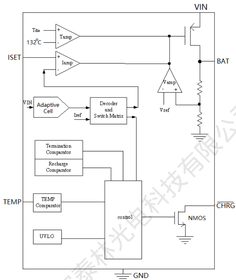
图 2 功能框图
