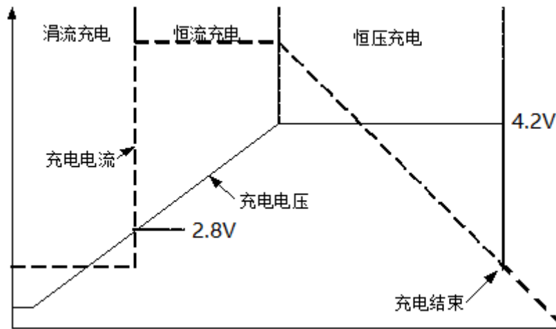
图3 充电过程示意图
